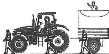
Wagenengel bei Traktoren mit zwei- oder einachsigen Hängern
